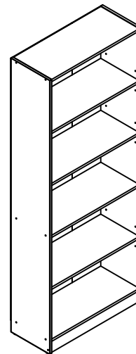
EDEN Item : EDEN BOEKENREK / ETAGERE Model : DN STC 201450 W700 x D295 x H1800mm
