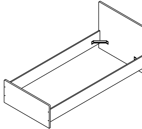
EDEN Item : EDEN BED90 Model : DN BED 3653 L2060 x W970 x H860mm
