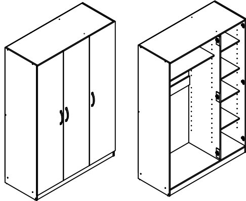
EDEN Item : EDEN KLEERKAST / GARDE ROBE 120 Model : DN WAR 300103 W1200 x D500 x H1800mm
